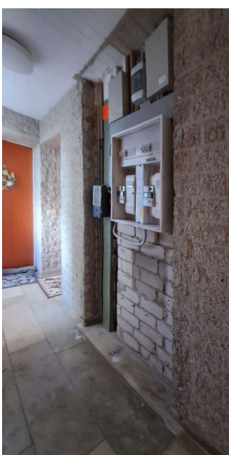
Schachtausbildung und Abschottung der elektrischen Verteileranlagen in den Fluren eines Seniorenheims
